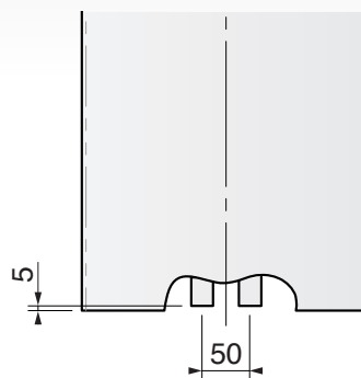
Kytkenämitat – vaihtoehto 5 & 6
